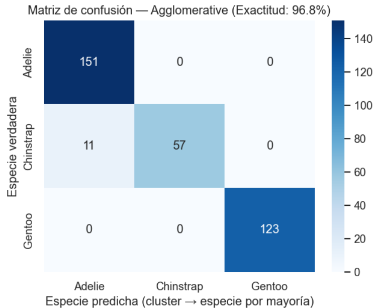
Figura 5: Matriz de confusión de Agglomerative Clustering (linkage=Ward) tras mapear cada cluster a su especie mayoritaria. Diagonal: aciertos; fila Chinstrap , columna Adelie : 11 ejemplares confundidos. Exactitud global: 96.8 %.
