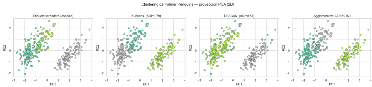
Figura 4: Proyección PCA 2D de las 342 observaciones. De izquierda a derecha: etiqueta verdadera de especie, K-Means, DBSCAN y Agglomerative. El ARI consignado en el título de cada panel corresponde al modelo correspondiente.
