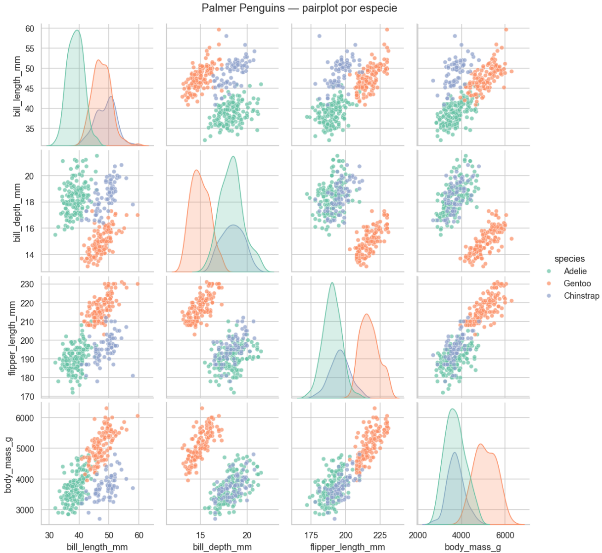
Figura 1: Pairplot de las cuatro variables morfométricas discriminado por especie. Gentoo se separa claramente del par Adelie/Chinstrap , especialmente en flipper_length_mm y body_mass_g . Adelie y Chinstrap comparten masa corporal y longitud de aleta similares, pero se distinguen por la longitud del pico.
