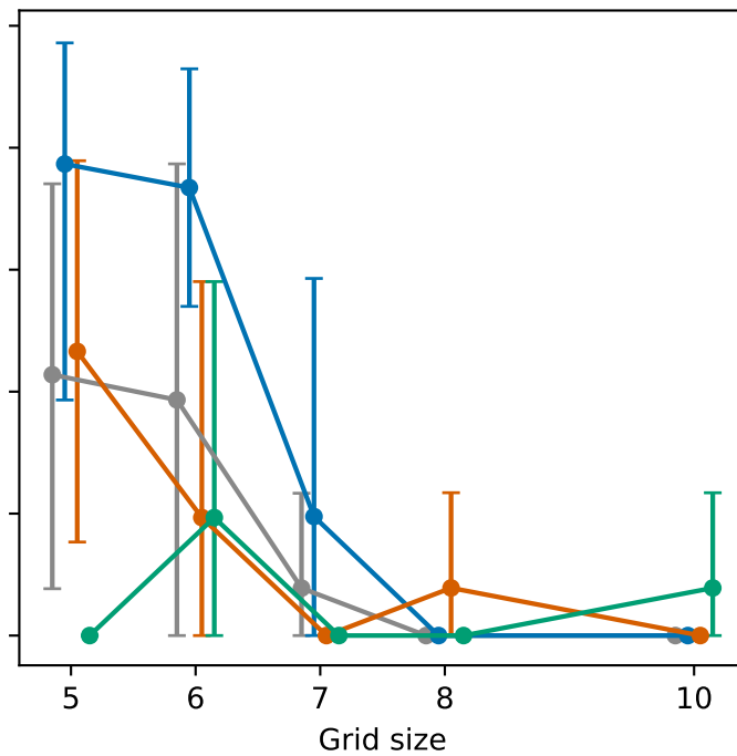
DoorKey
