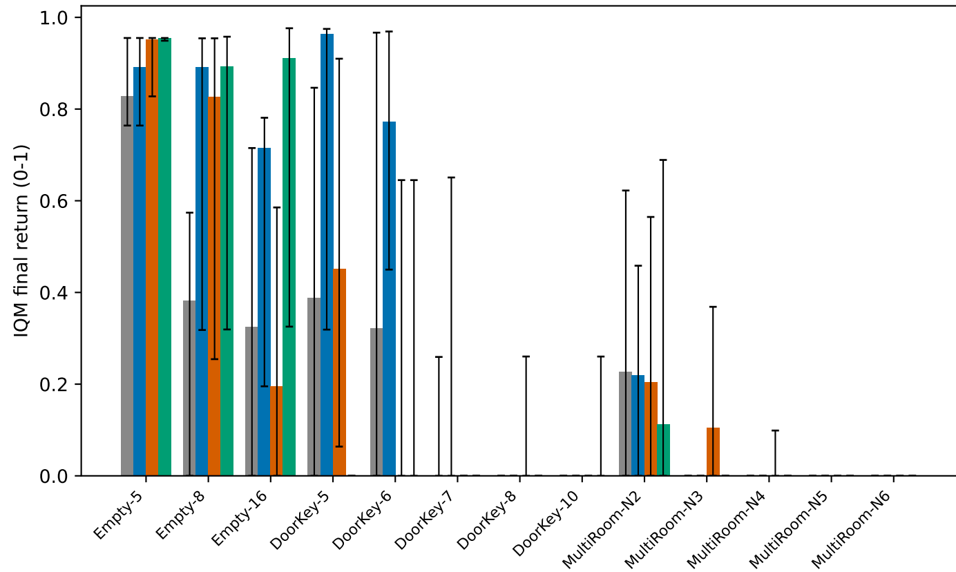
Per instance
