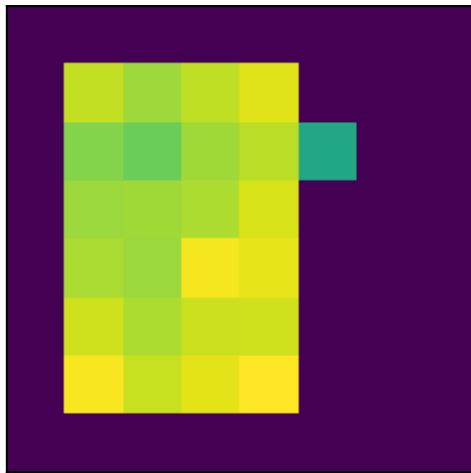
\epsilon -greedy
