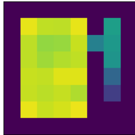
NoisyNets
