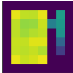
NoisyNets
