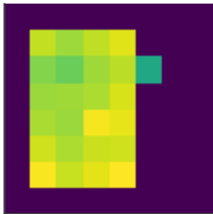
\epsilon -greedy
