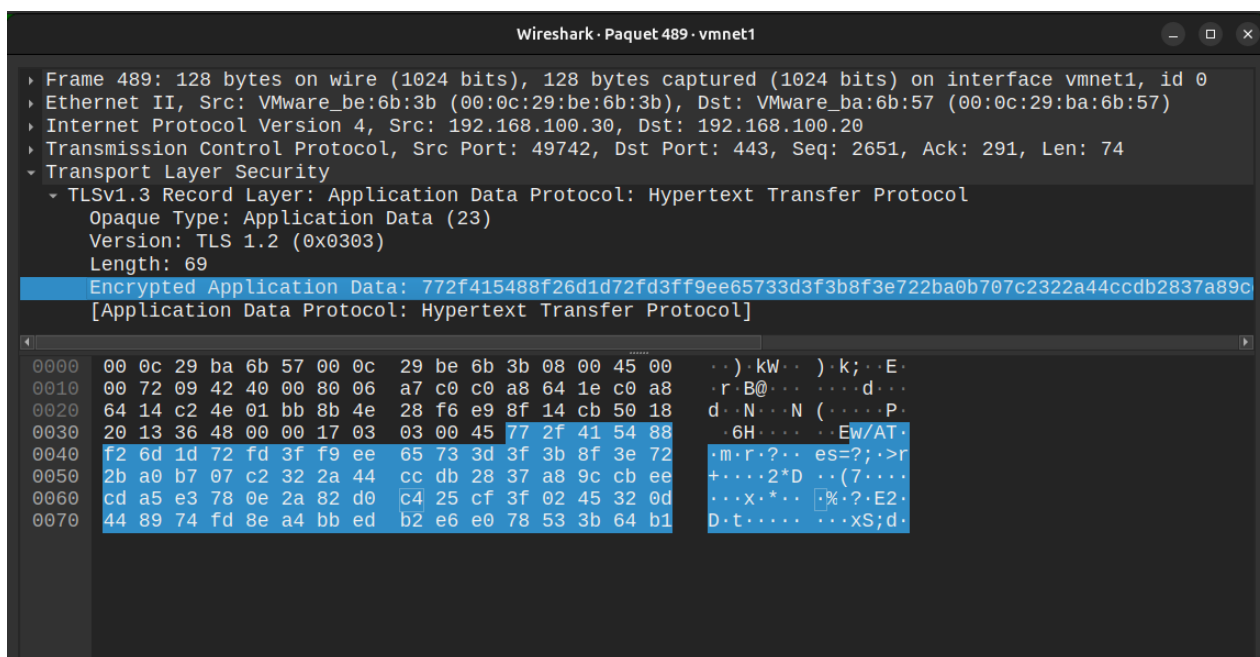
Figure 118 : Analyse d'un échange TLS dans Wireshark.
