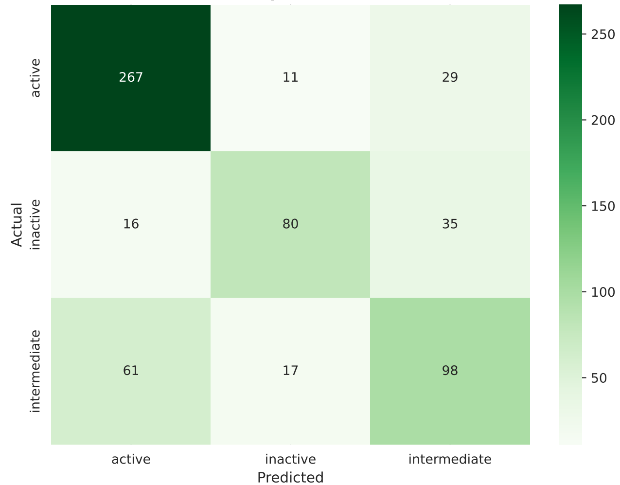
TopK-512
