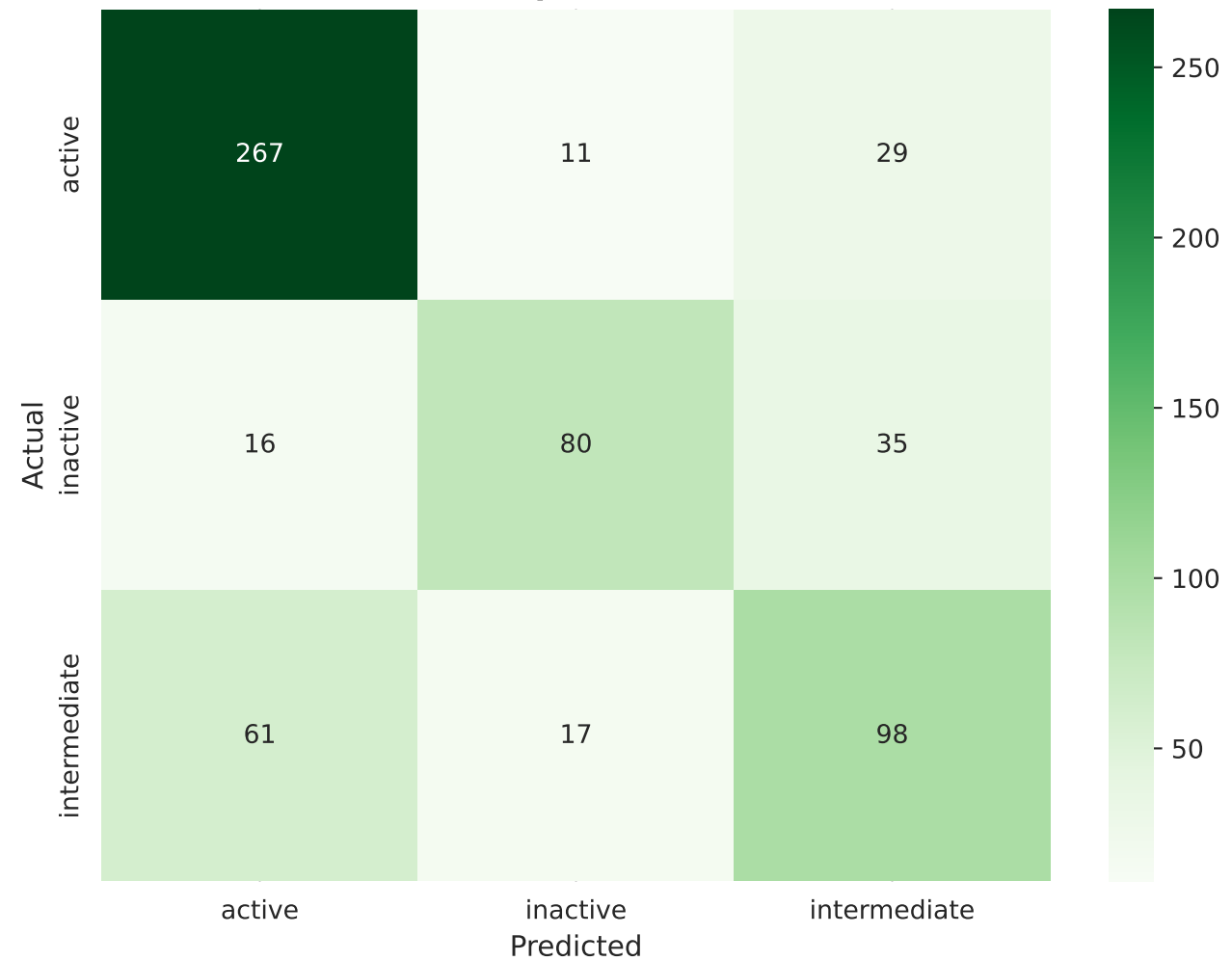
TopK-512
