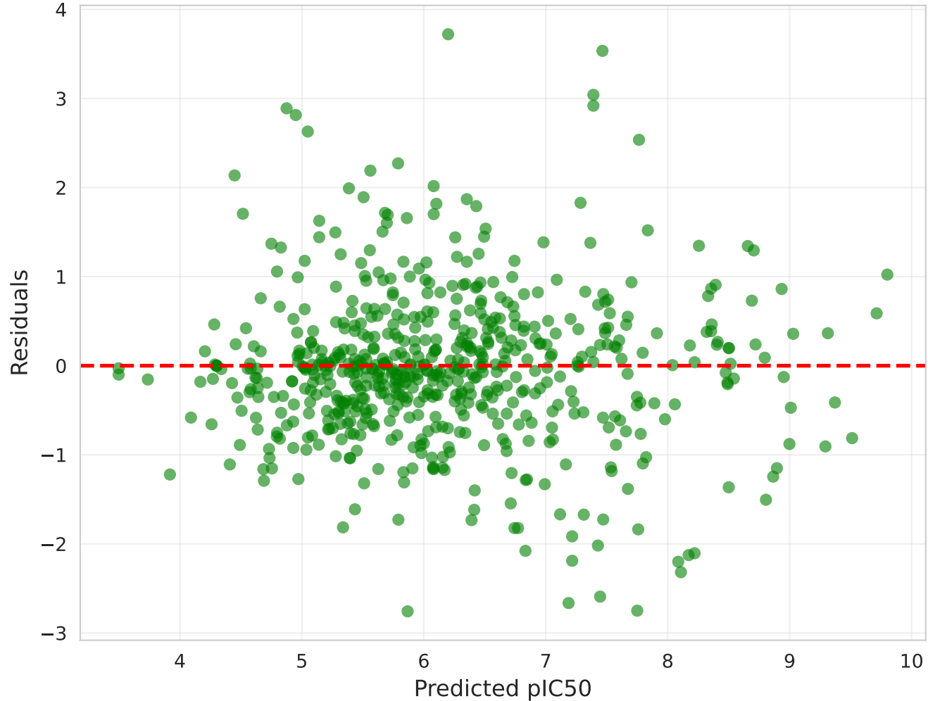
TopK-512 (RMSE=0.850)
