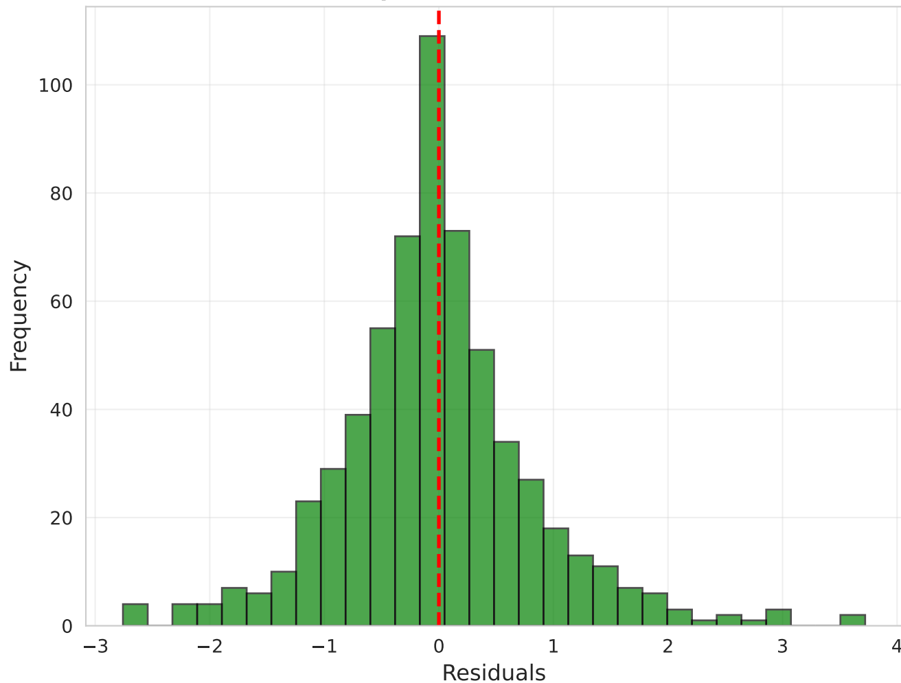
TopK-512 (MAE=0.606)
