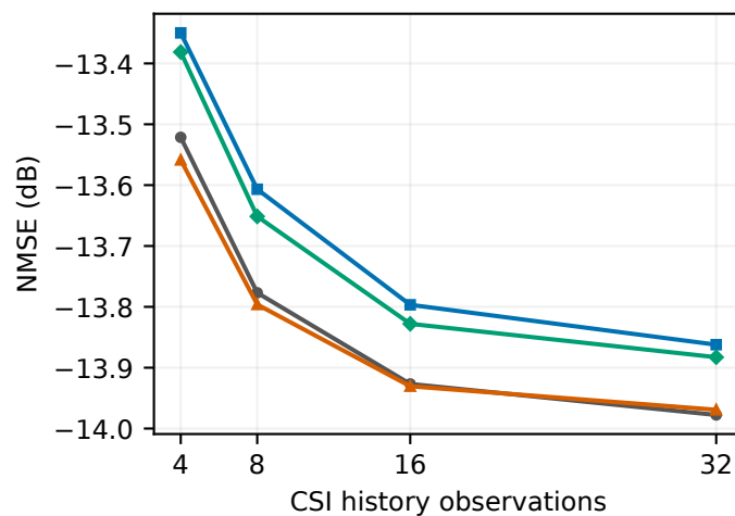
Far LoS
