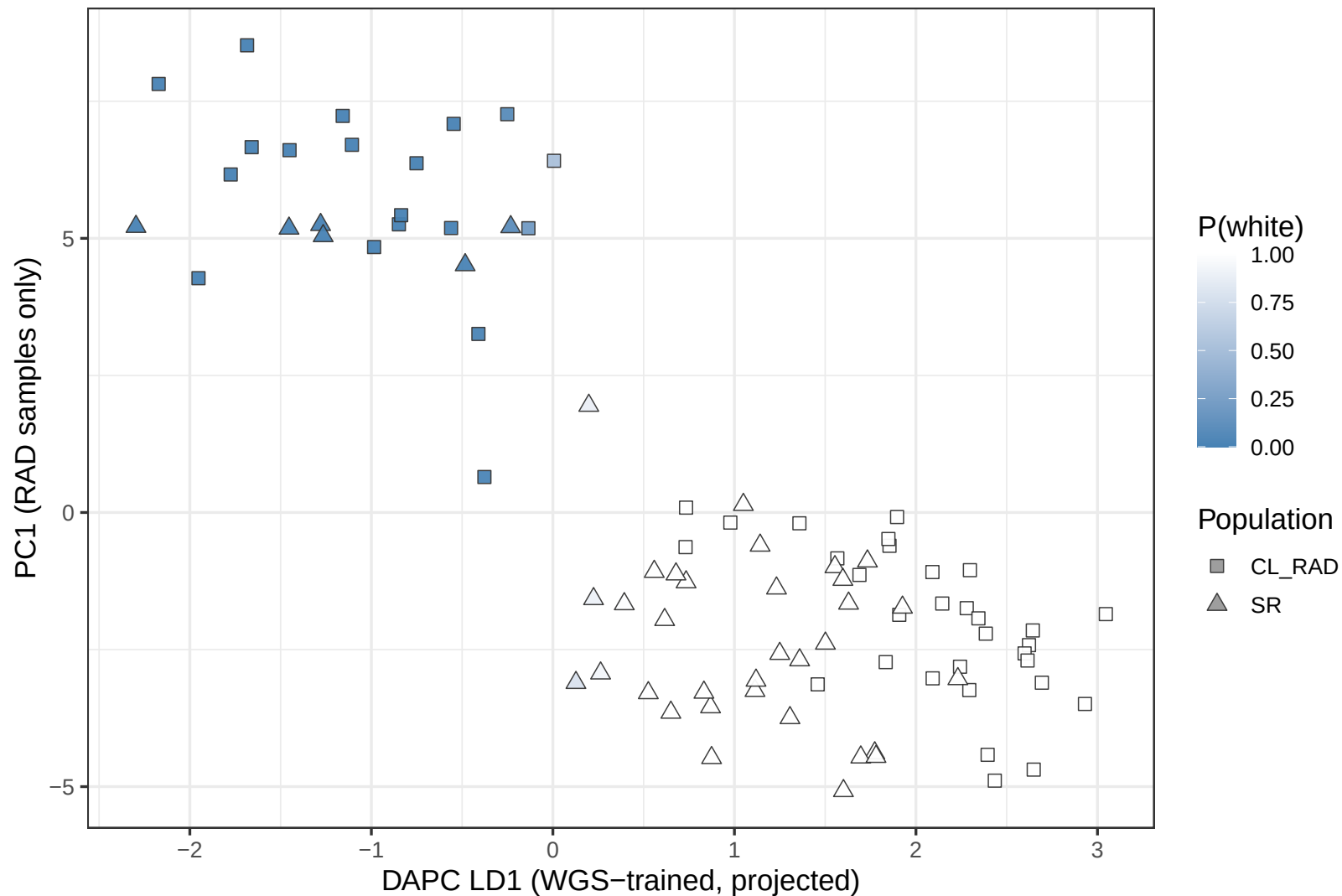
RAD-only: DAPC LD1 vs RAD-subset PC1
