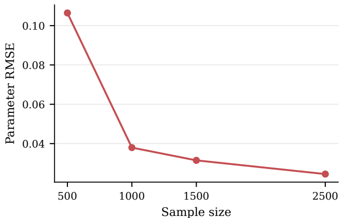
(c) Gamma--lognormal parameter accuracy
