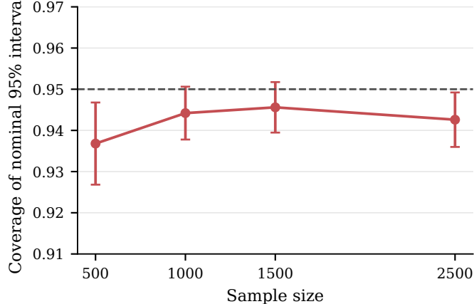
(d) Gamma--lognormal Wald coverage
