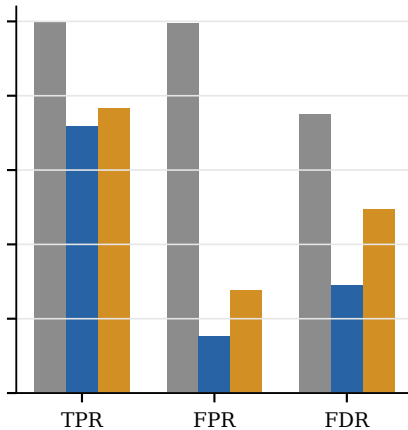
Gamma-lognormal
