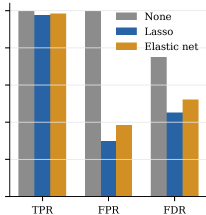
Poisson--ZIP
