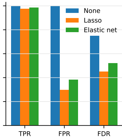
Poisson--ZIP
