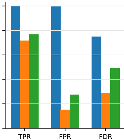
Gamma--lognormal
