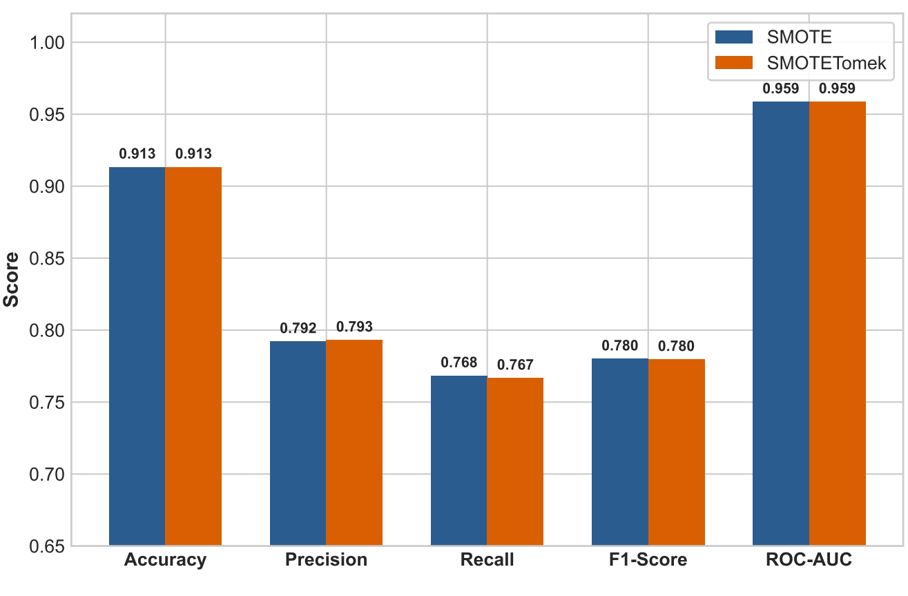
(D) Key Metrics Summary (SMOTE vs SMOTETomek)
