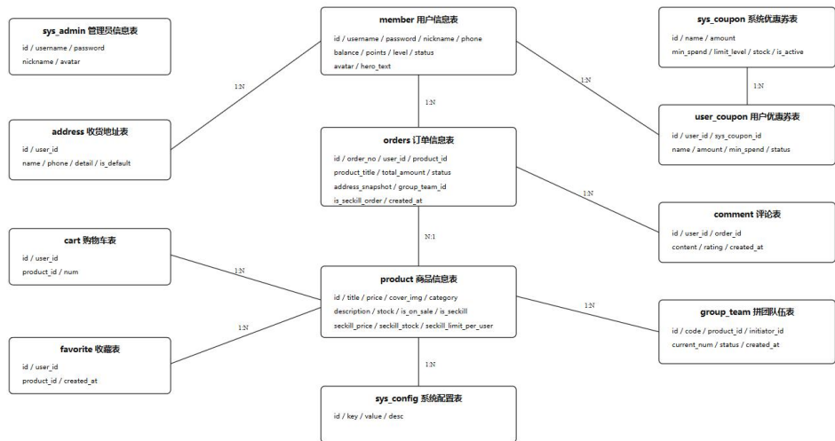
图 3.3 系统 E-R 图
