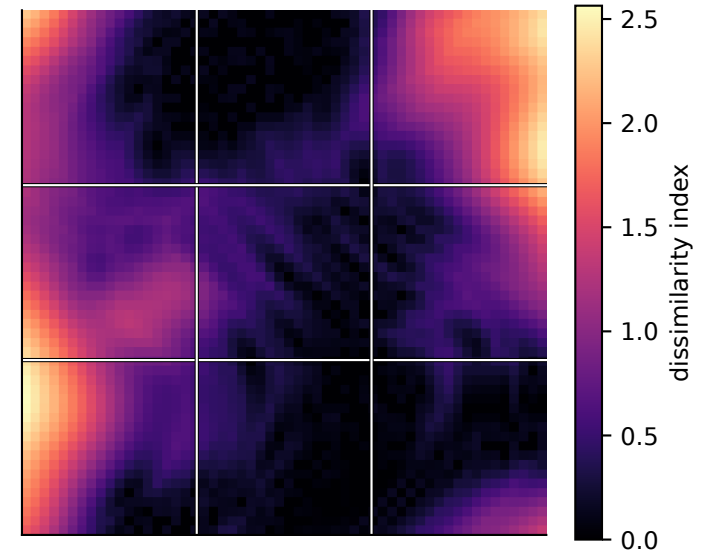
(d) dissimilarity index for the design in (a)
