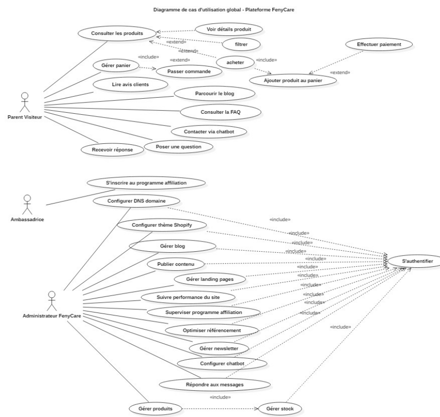
FIGURE 3.1 – Diagramme de cas d'utilisation f de la plateforme FenyCare
