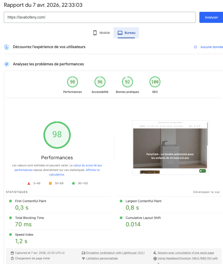
FIGURE 6.1 – Résultats PageSpeed Insights — Version Bureau
