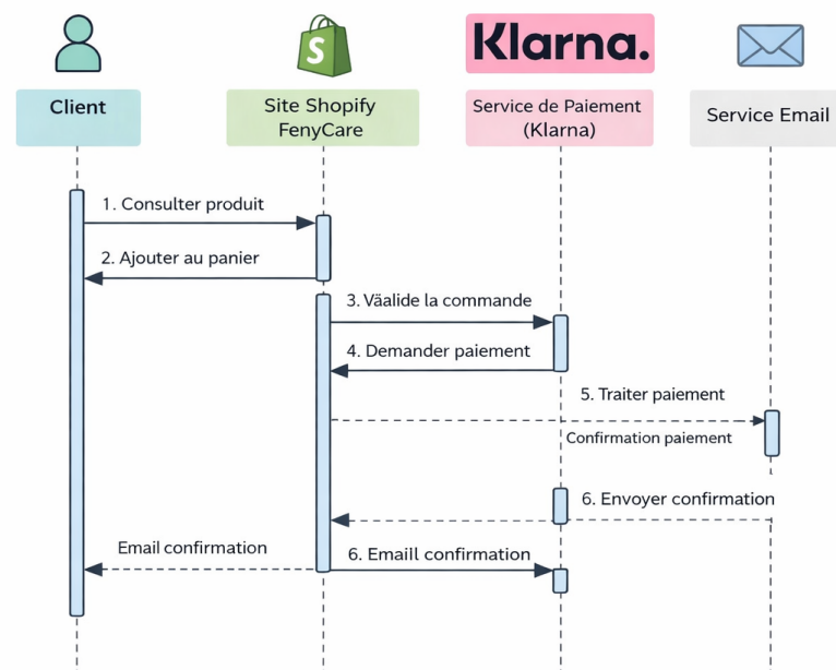
Diagramme de séquence du parcours d'achat
