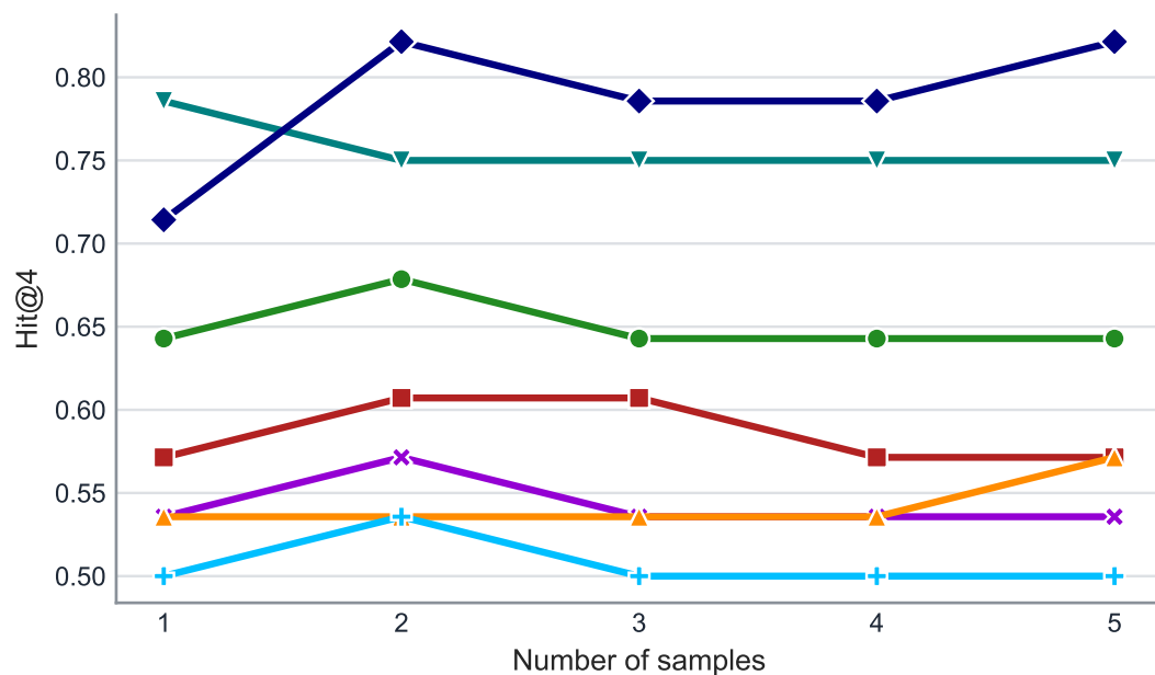
Hit@4
