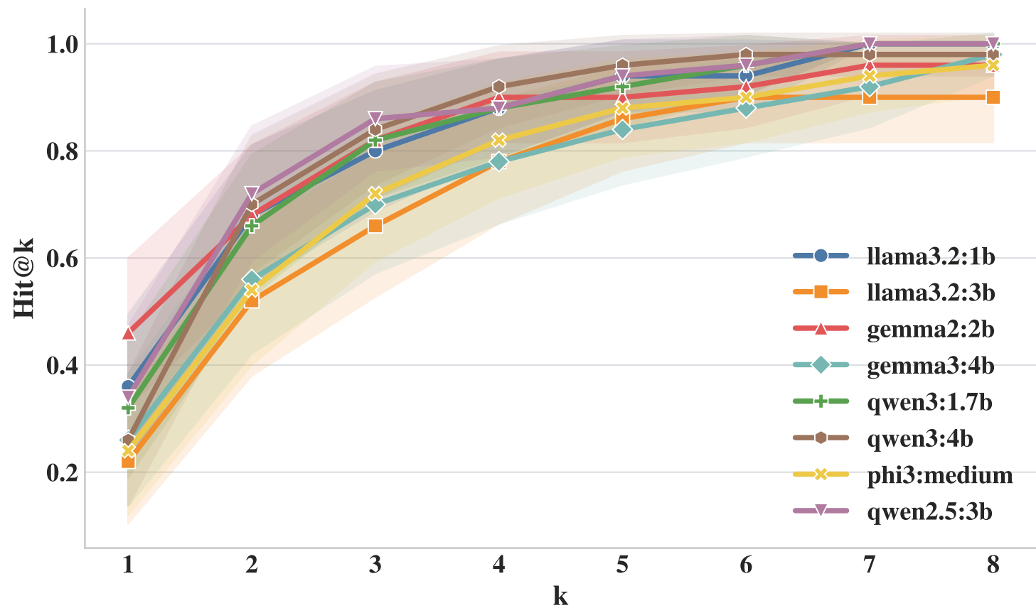
Hit@k
