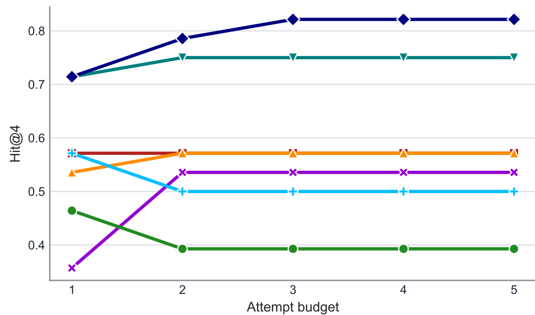
Hit@4
