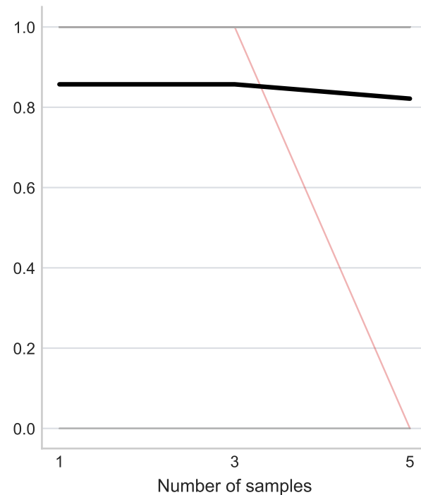
Hit@4
