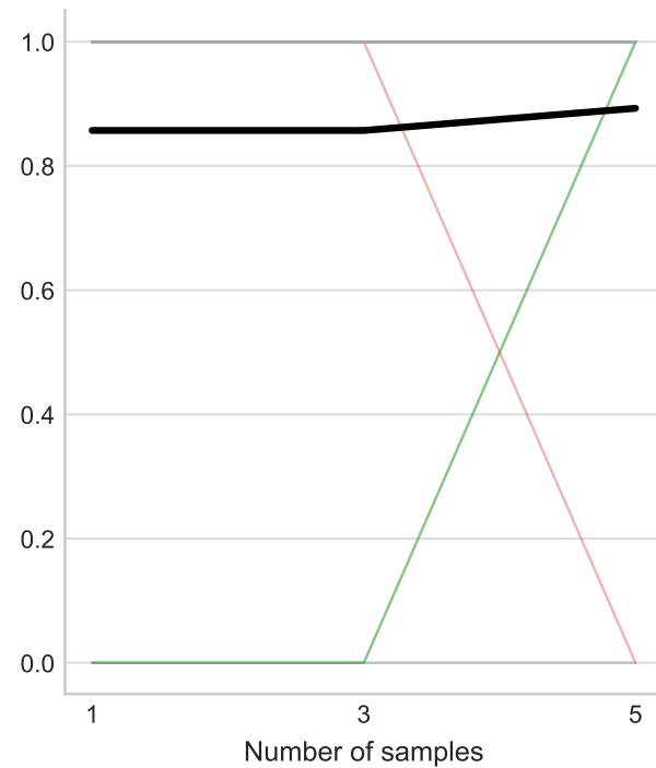
Hit@4
