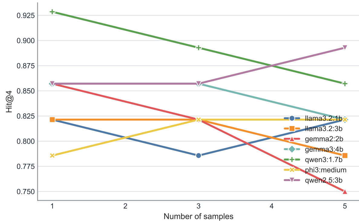
Hit@4
