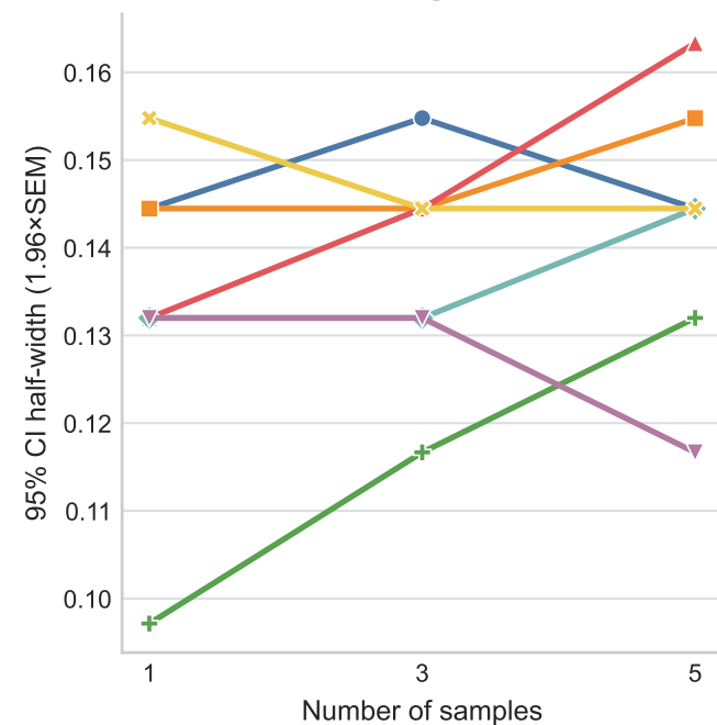
Hit@4
