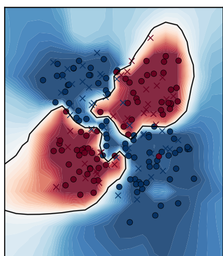
XOR
