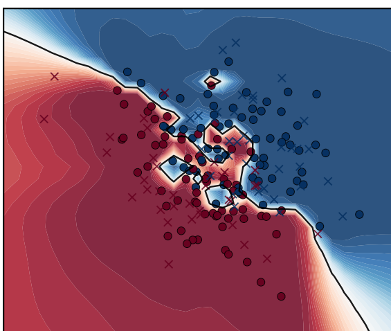
Anisotropic Blobs
