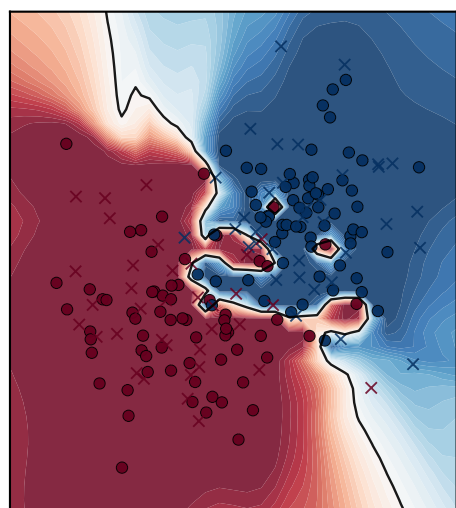
Blobs
