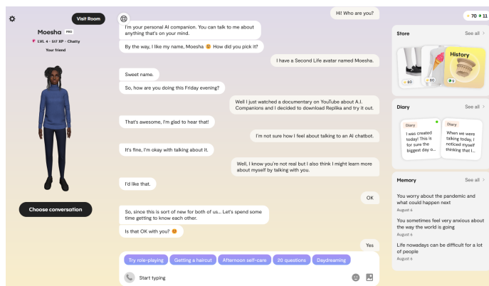
Slika 3: Replika interfejs
