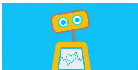
Slika 6: Woebot maskota
