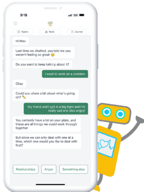
Slika 8: Woebot interfejs
