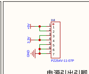
电源引出引脚
