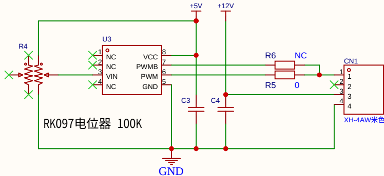
PWM输出电路
