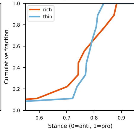
(d) NLI Stance CDF (ai_conference)
