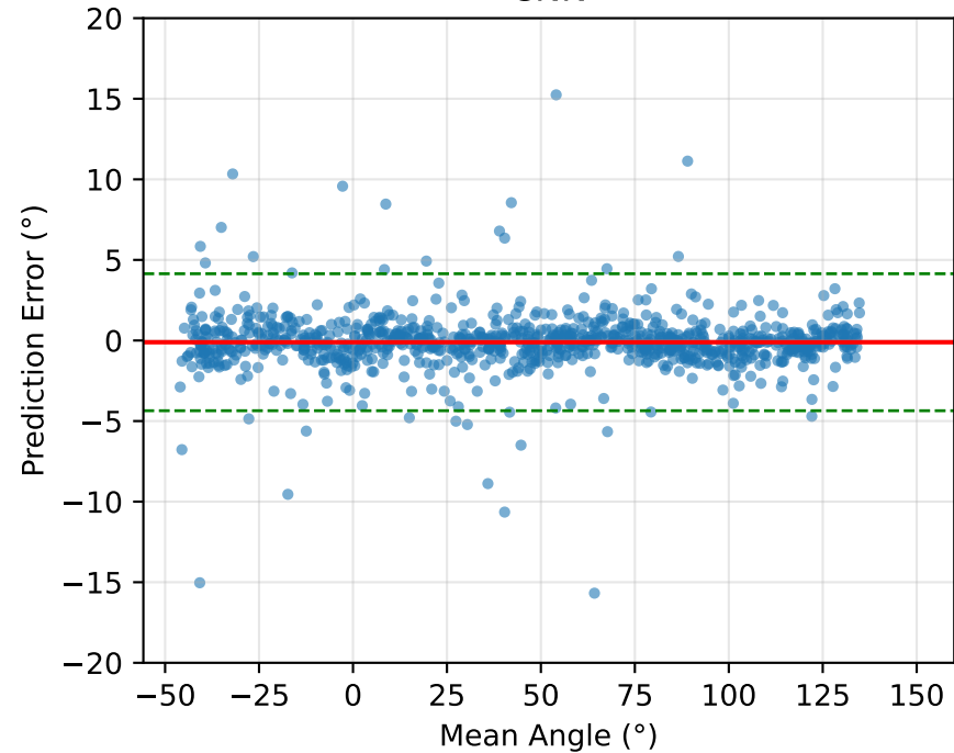
CNN
