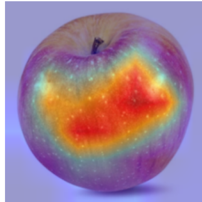
MobileNetV2
