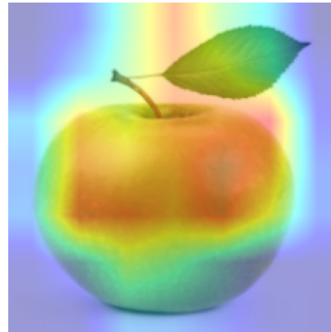
MobileNetV2
