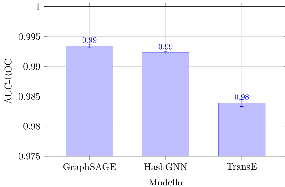
Figura 4.2: AUC-ROC medio con deviazione standard per i tre modelli su 5 run indipendenti
