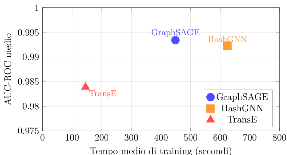
Figura 4.4: Trade-off tra accuratezza (AUC-ROC) ed efficienza computazionale
