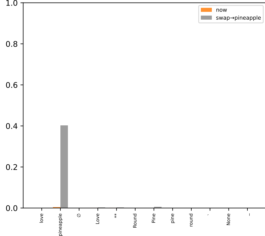
QwenInst: love KL=1.62
