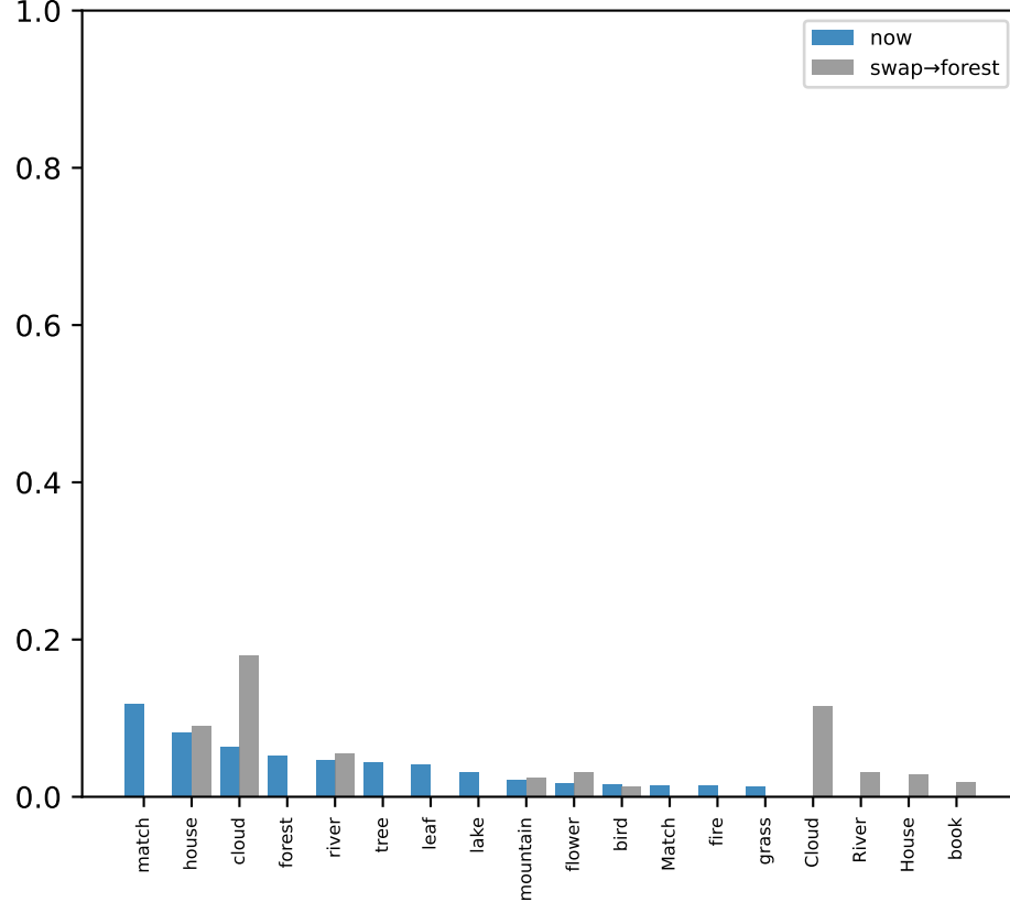
LlamaInst: river KL=0.68
