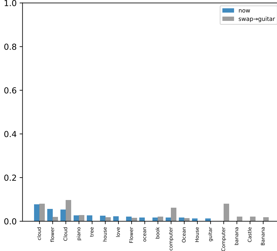
LlamaInst: ocean KL=0.34
