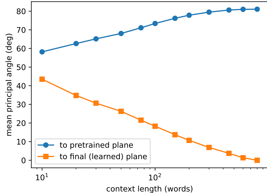
subspace trajectory
