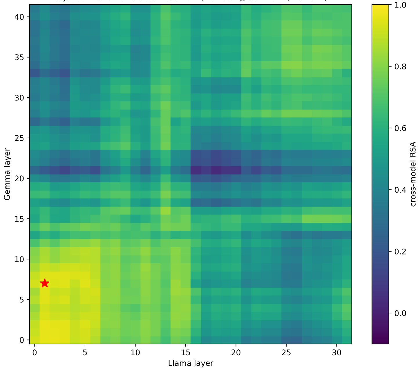
days: Gemma vs Llama cross-model RSA (max 0.97 @ Gemma L7 / Llama L1)
