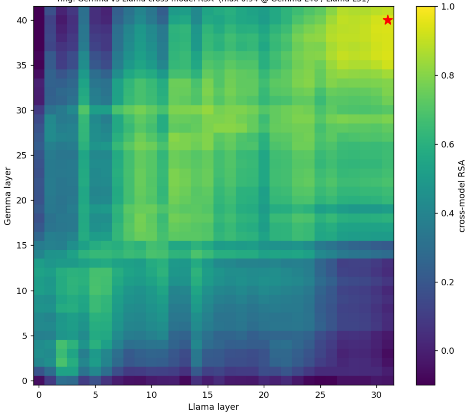
ring: Gemma vs Llama cross-model RSA (max 0.94 @ Gemma L40 / Llama L31)
