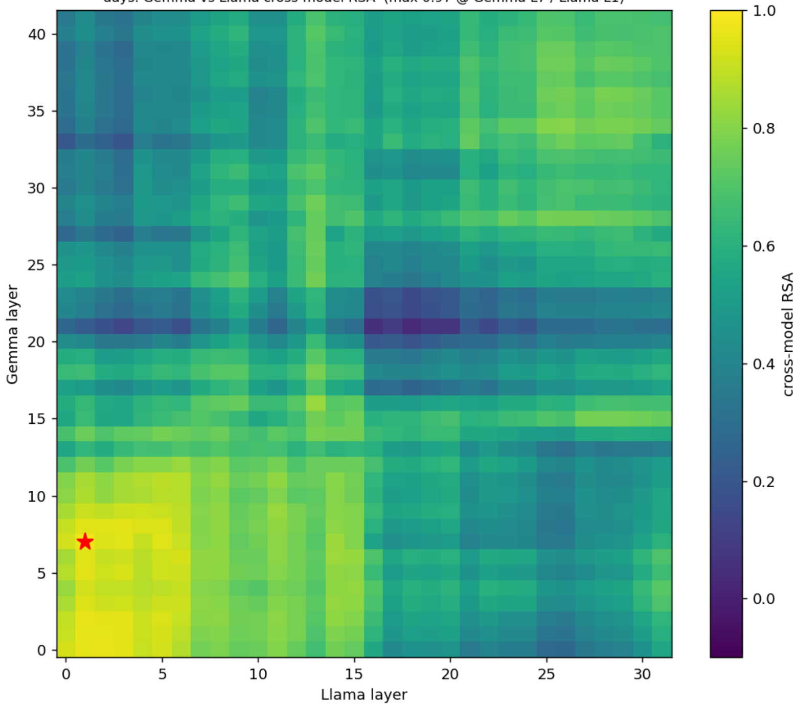
days: Gemma vs Llama cross-model RSA (max 0.97 @ Gemma L7 / Llama L1)
