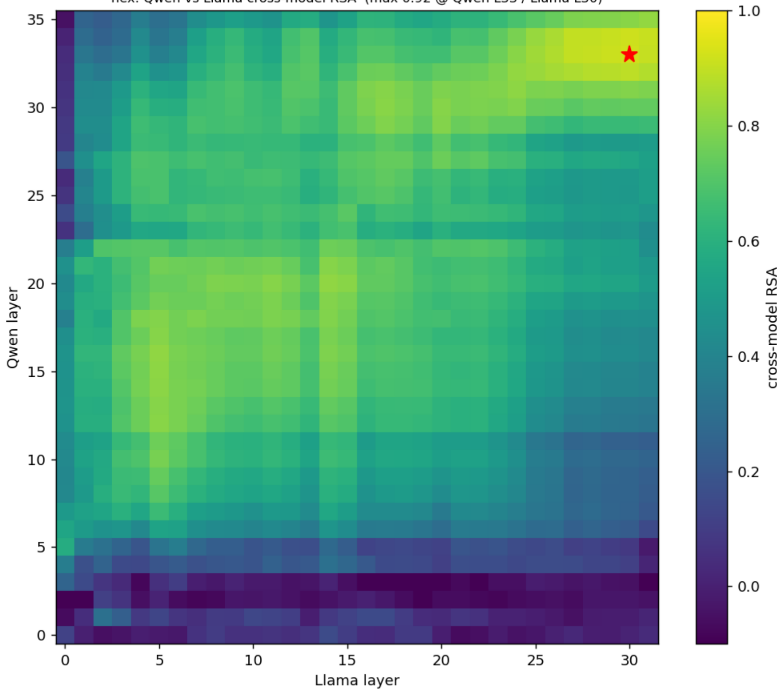
hex: Qwen vs Llama cross-model RSA (max 0.92 @ Qwen L33 / Llama L30)
