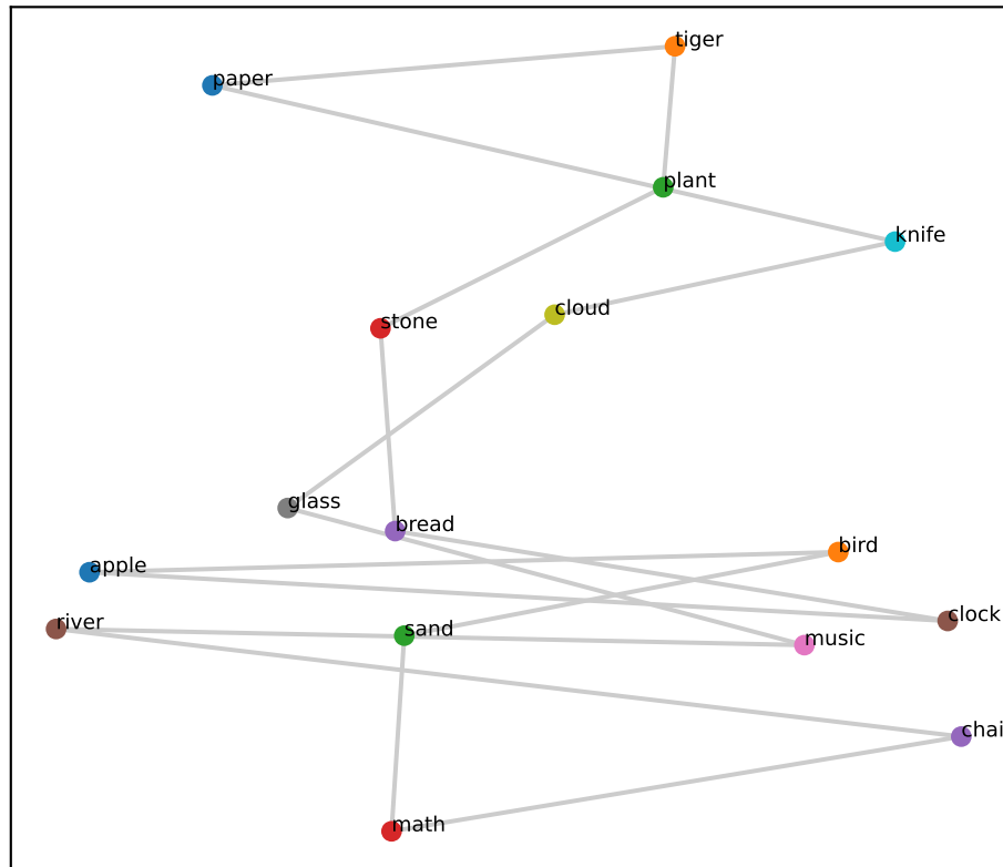
Llama L19 (RSA=+0.42)
