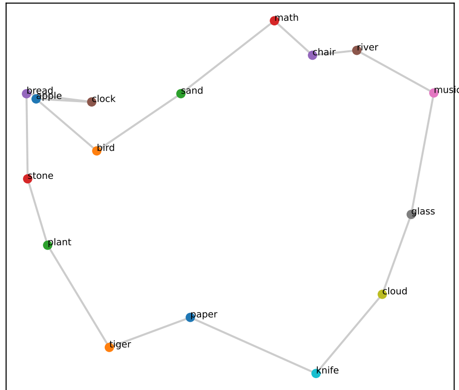
Gemma L27 (RSA=+0.66)
