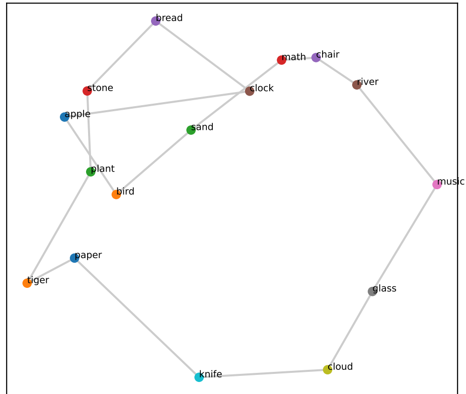
Gemma L16 (RSA=+0.41)
