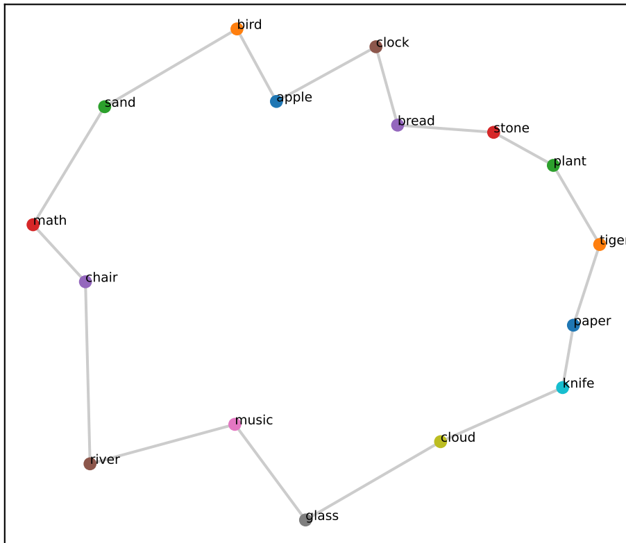
Llama L25 (RSA=+0.72)
