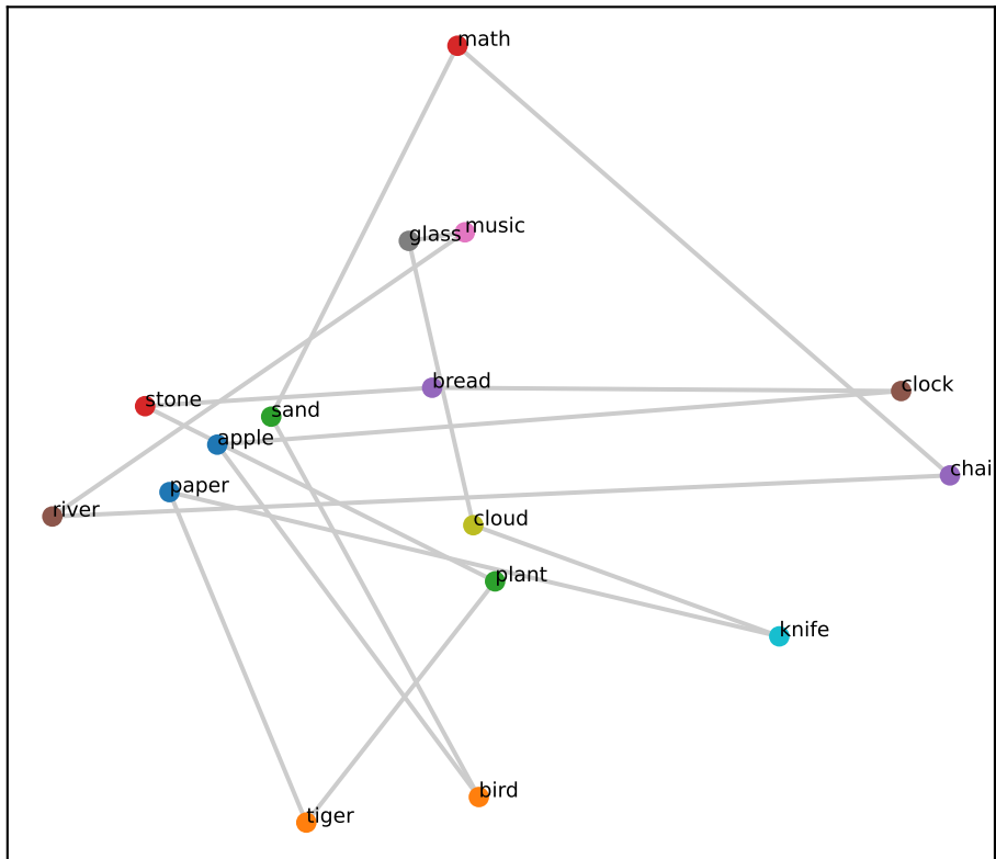
Llama L6 (RSA=+0.02)
