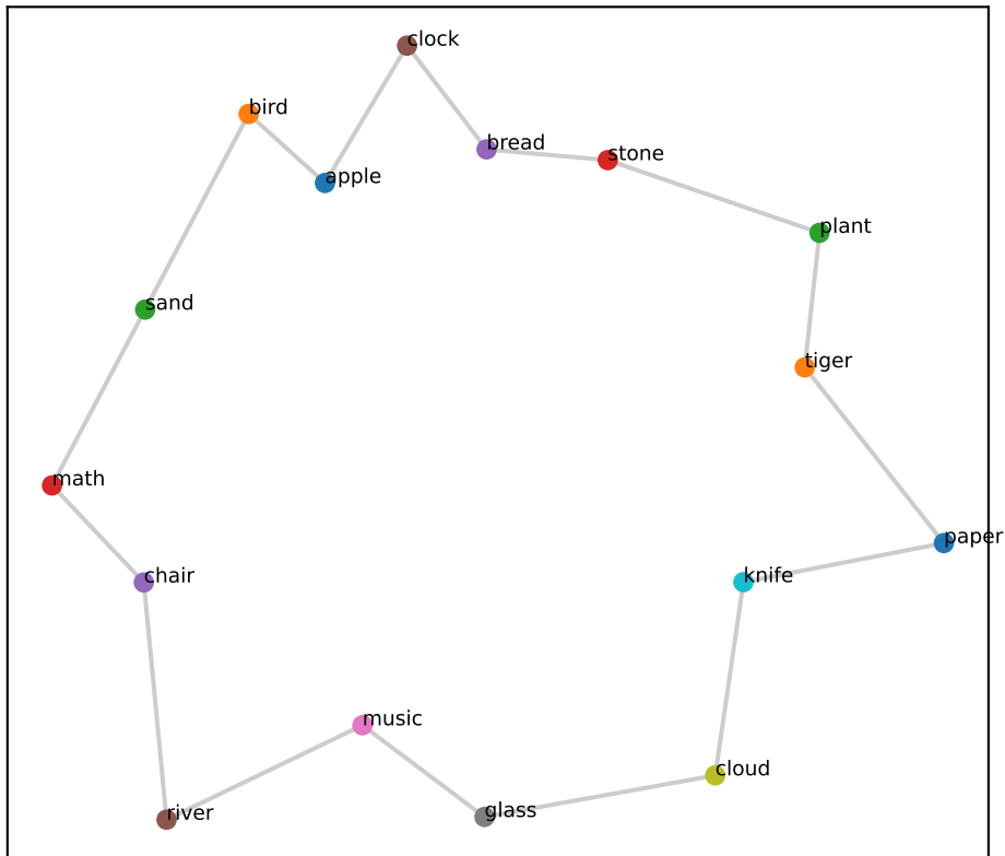
Llama L27 (RSA=+0.74)
