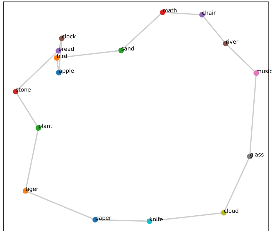
Gemma L28 (RSA=+0.54)
