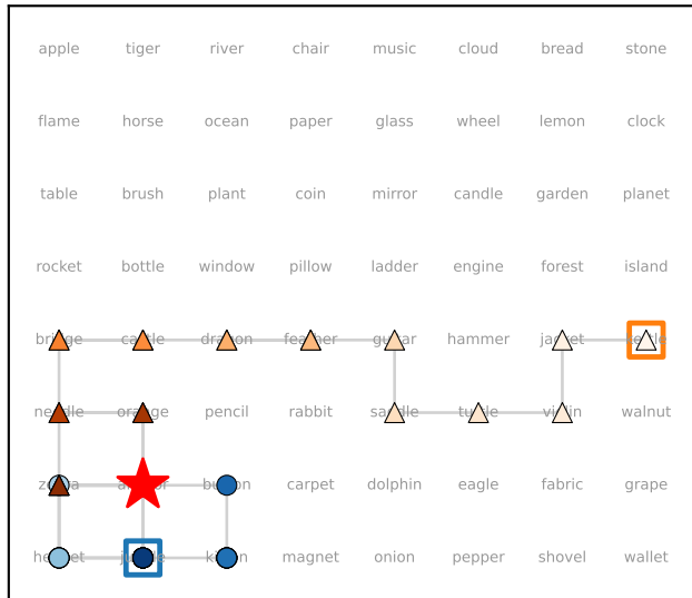
game 6: MET @r48
