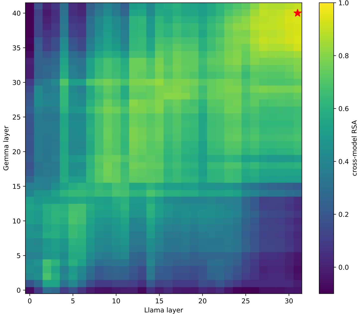
ring: Gemma vs Llama cross-model RSA (max 0.94 @ Gemma L40 / Llama L31)
