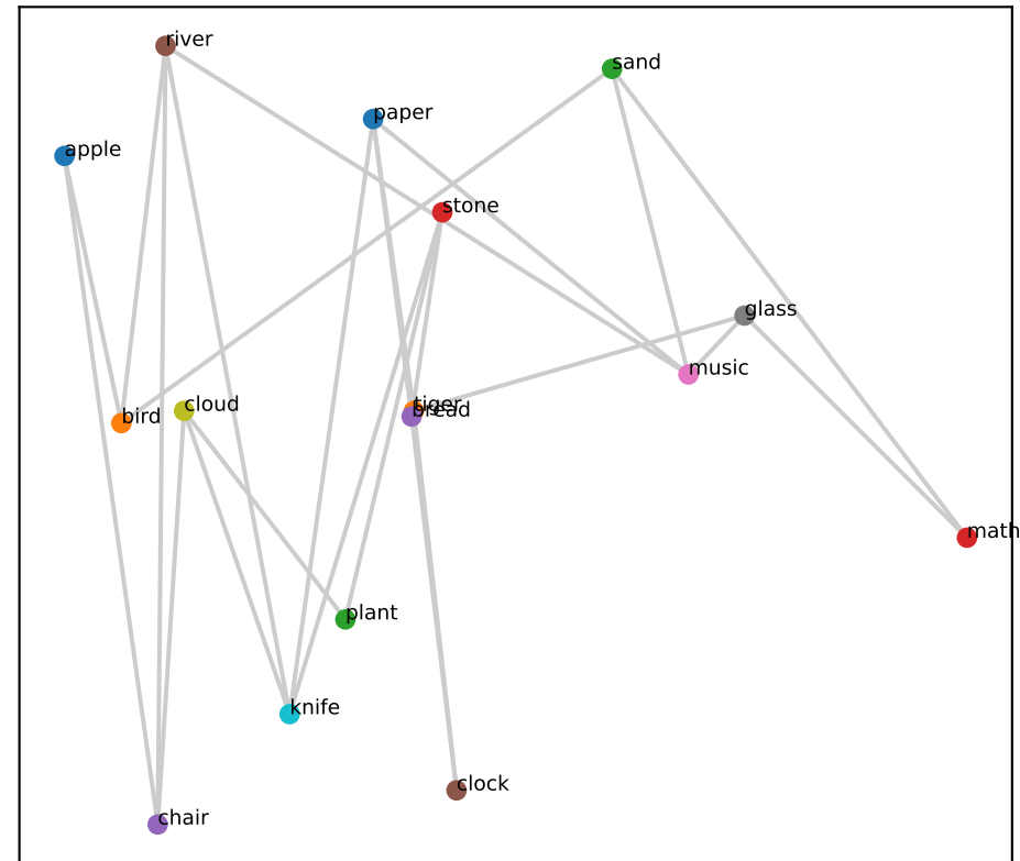
Llama L9 (RSA=0.46)
