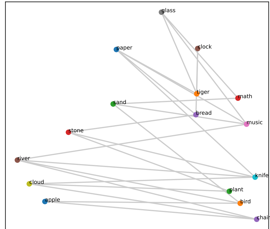
Llama L27 (RSA=0.37)
