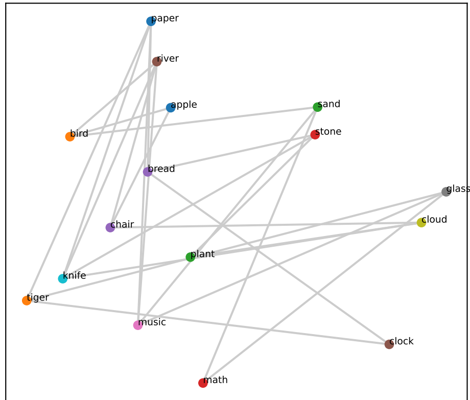
Qwen L18 (RSA=0.22)
