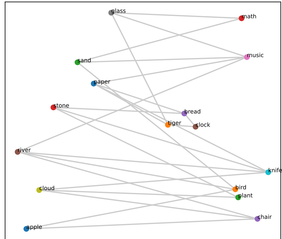
Llama L19 (RSA=0.24)
