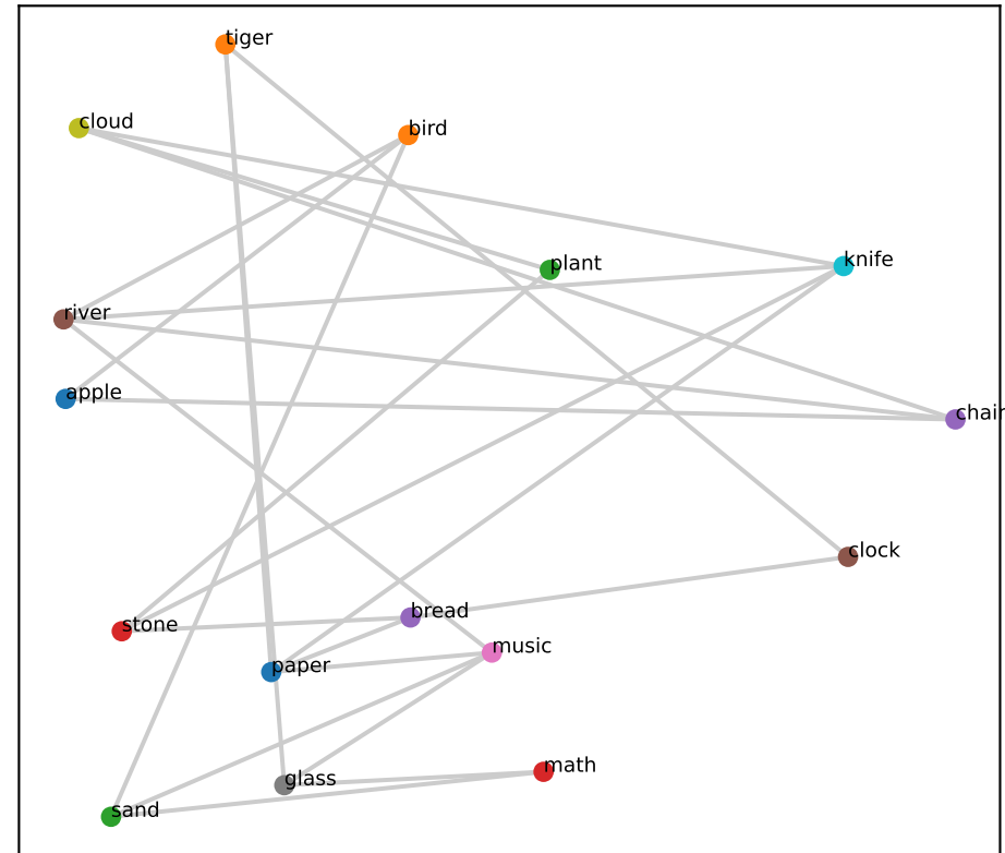
Llama L2 (RSA=0.17)
