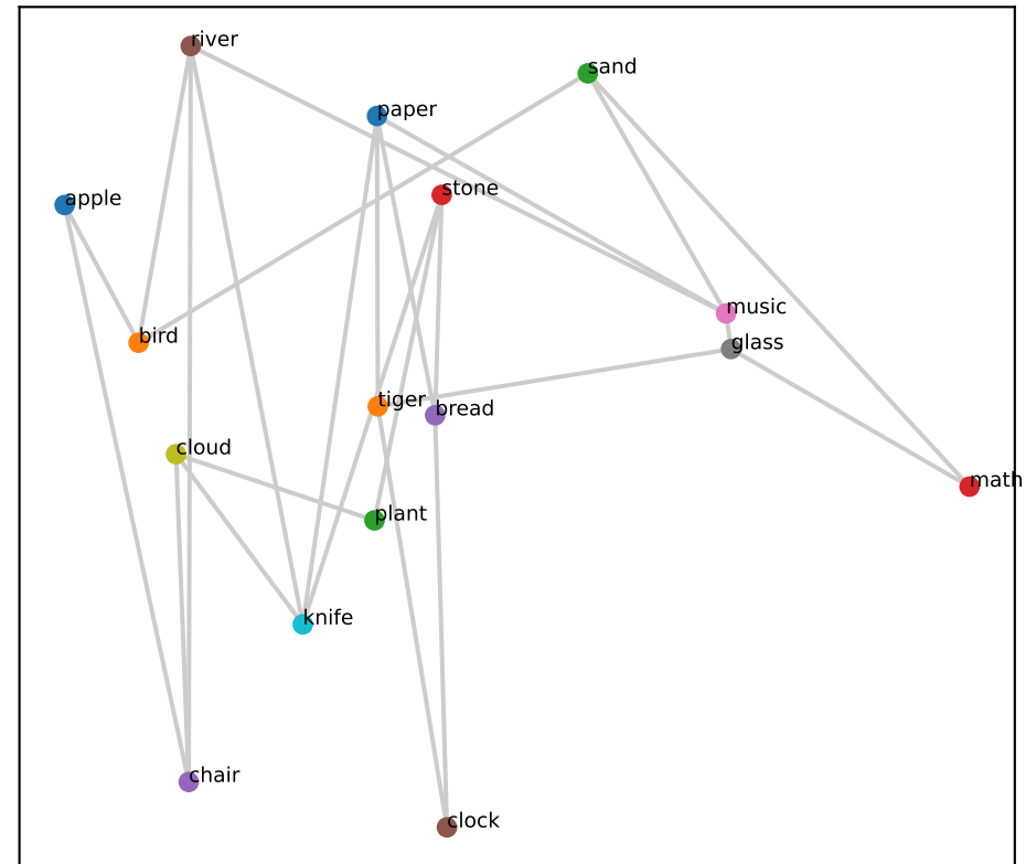
Llama L8 (RSA=0.42)
