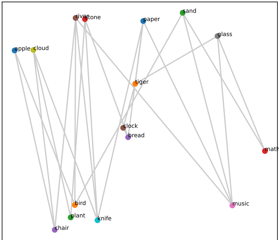
Gemma L30 (RSA=0.38)
