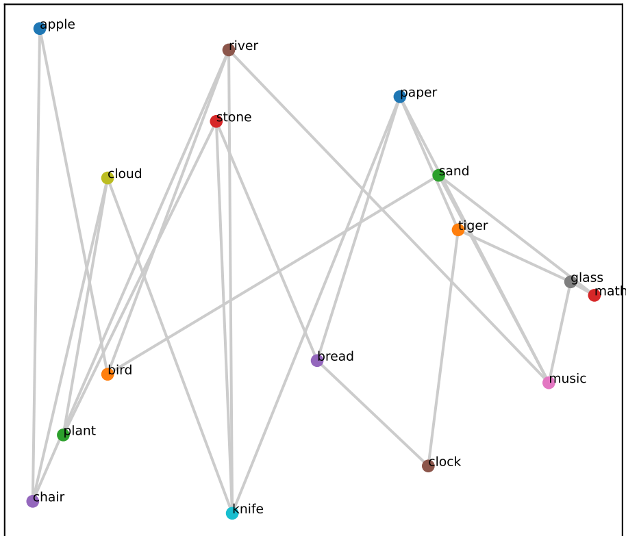
Gemma L24 (RSA=0.50)
