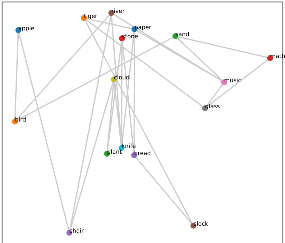
Gemma L15 (RSA=0.28)
