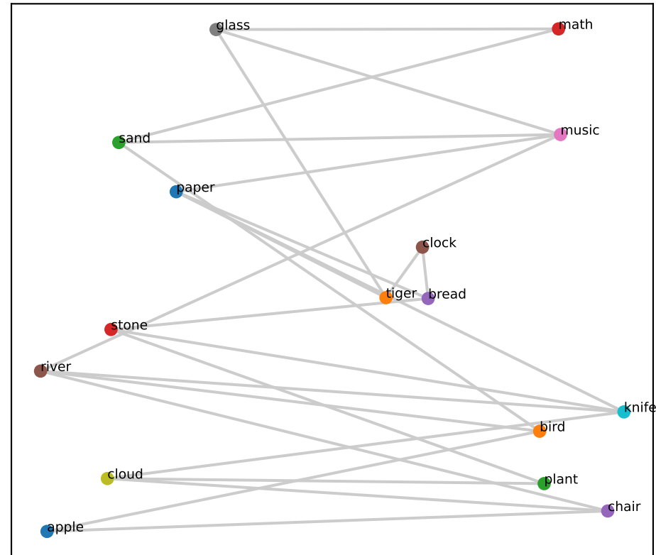
Llama L21 (RSA=0.32)
