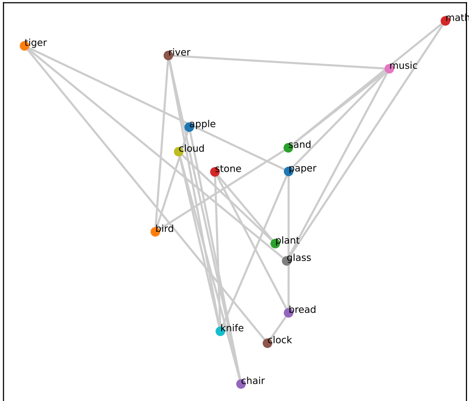
Gemma L10 (RSA=0.08)
