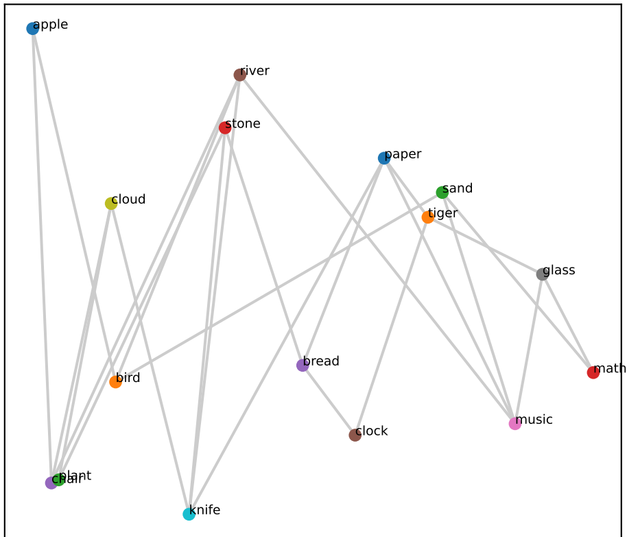
Gemma L27 (RSA=0.49)
