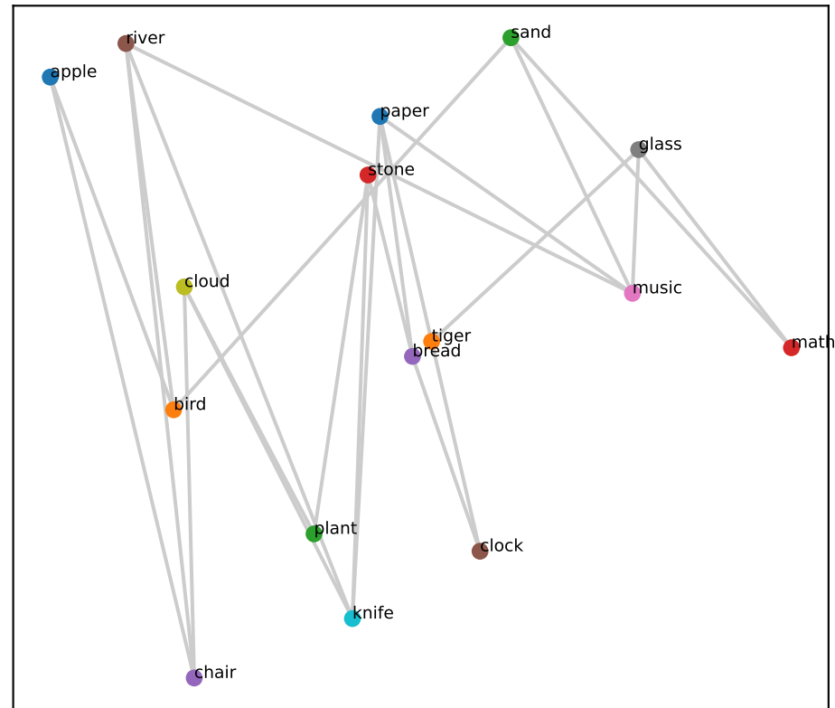
Llama L13 (RSA=0.54)
