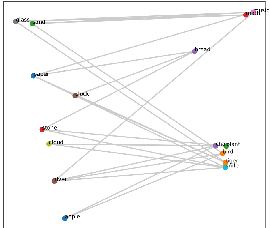
Qwen L23 (RSA=0.07)
