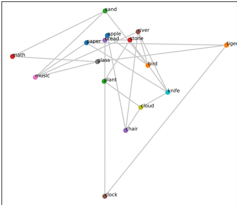
Gemma L4 (RSA=0.05)
