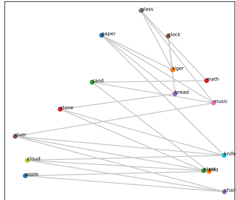
Llama L29 (RSA=0.43)
