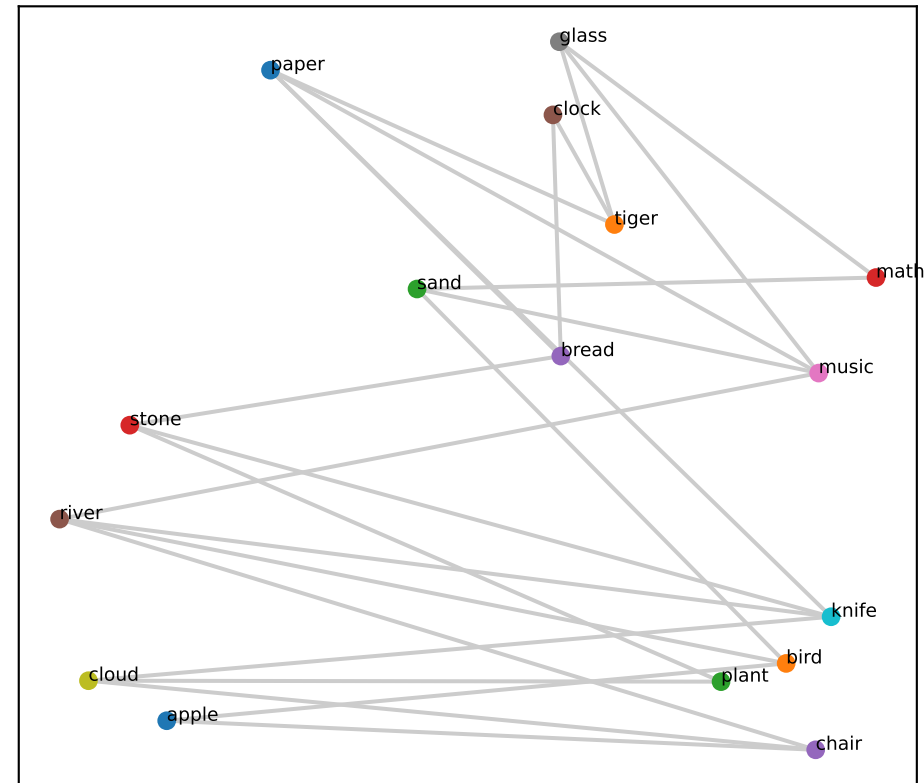
Llama L31 (RSA=0.31)
