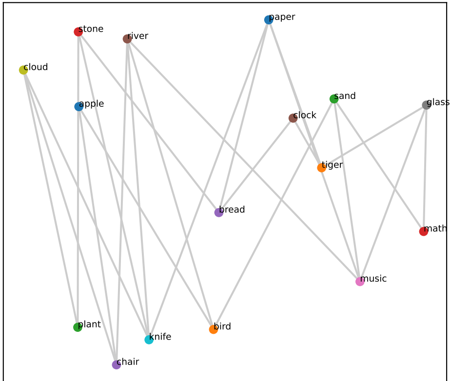
Gemma L39 (RSA=0.70)
