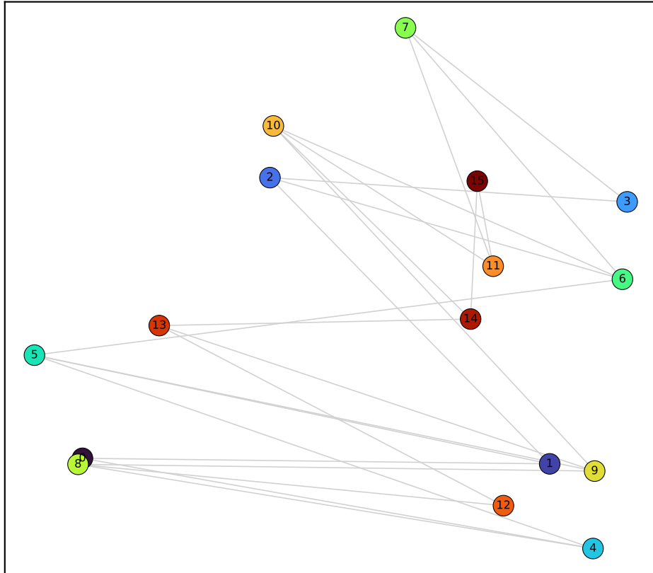
Llama layer 29/31 (PC var 20·16%)
