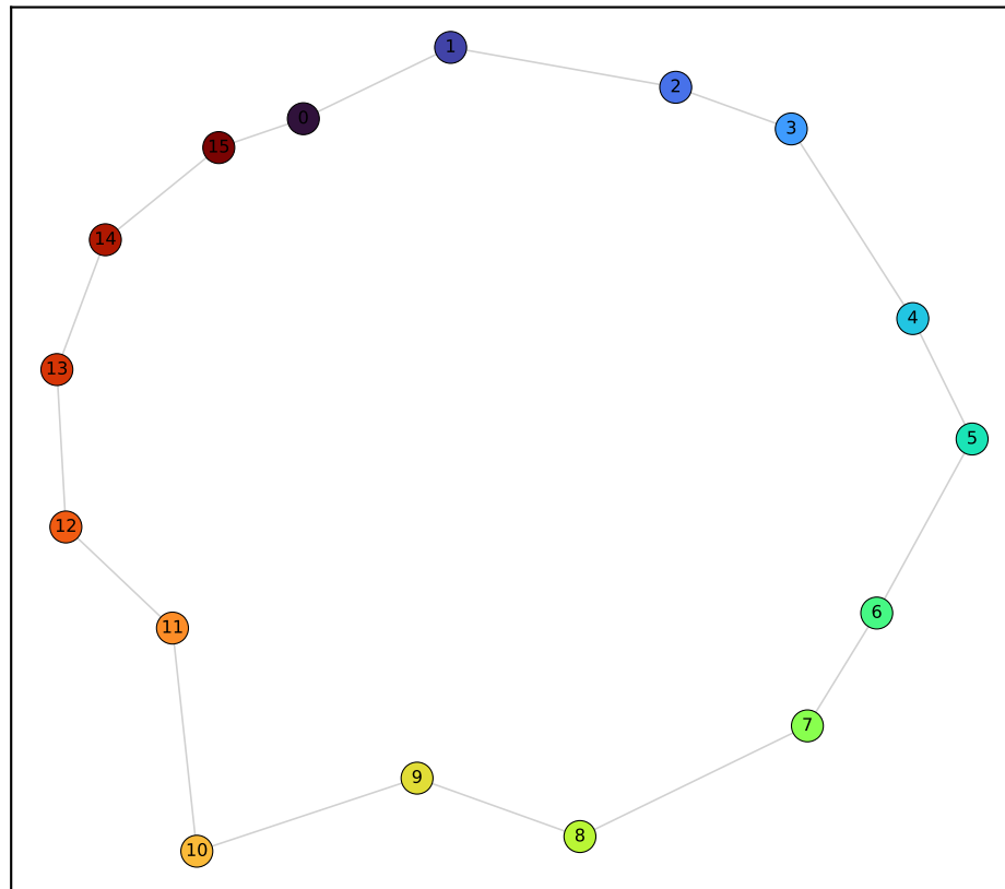
Gemma layer 39/41 (PC var 24·19%)
