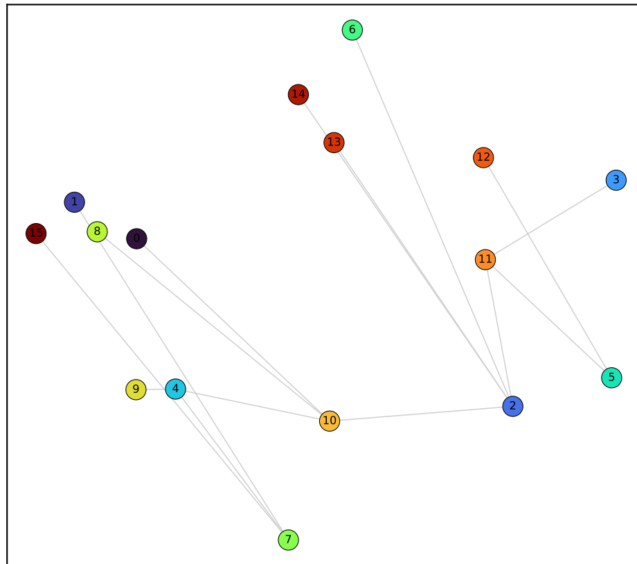
Gemma layer 27/41 (PC var 15·13%)
