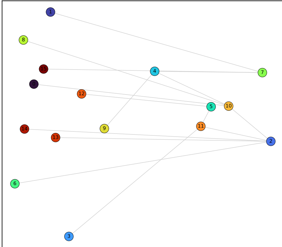
Llama layer 11/31 (PC var 22.9%)
