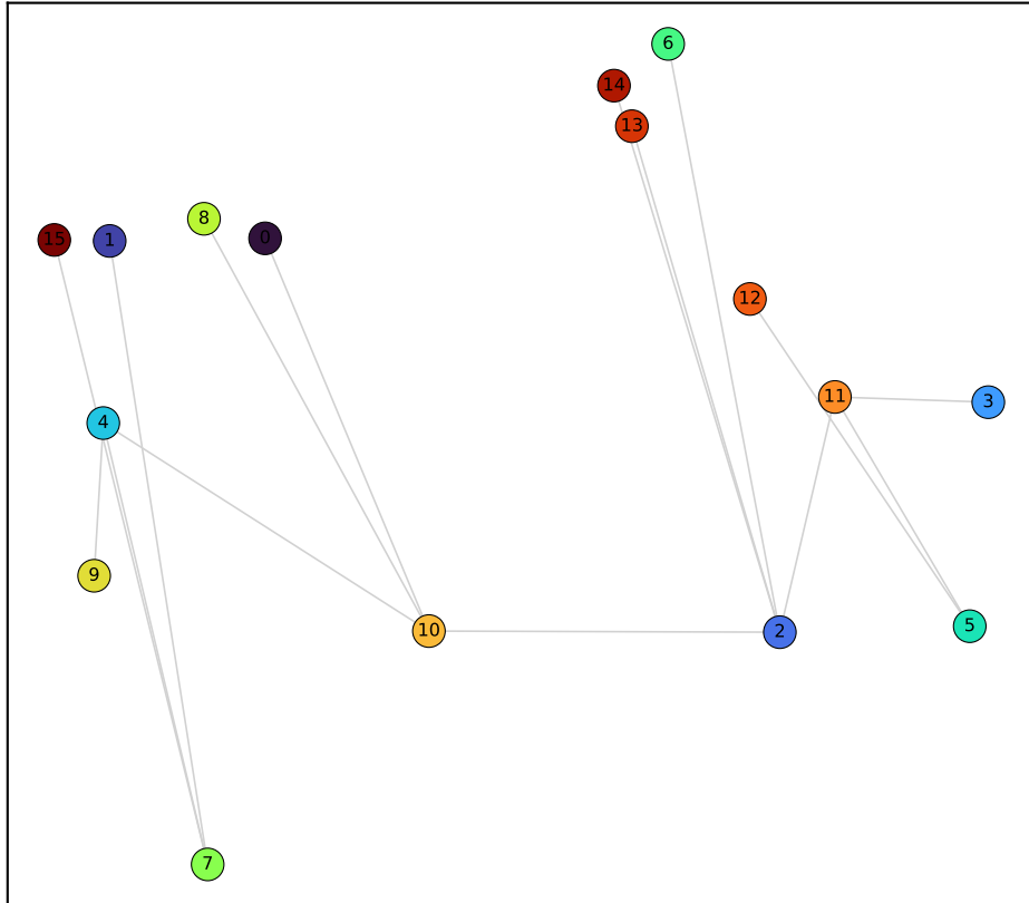
Llama layer 27/31 (PC var 19·17%)
