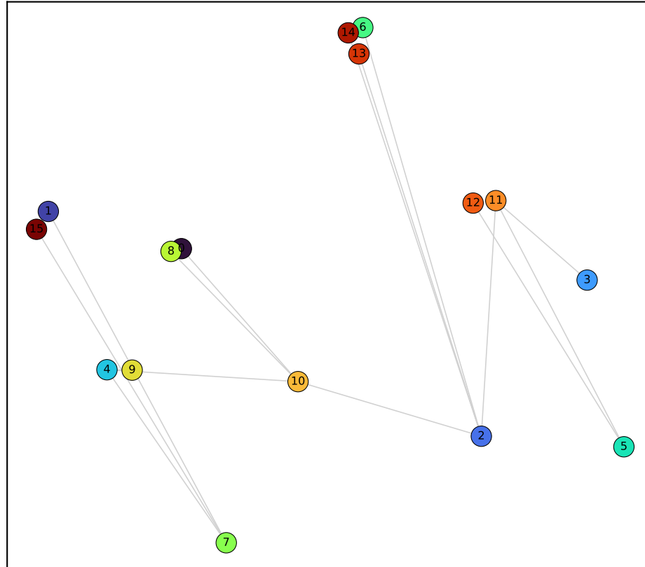
Gemma layer 36/41 (PC var 19·16%)
