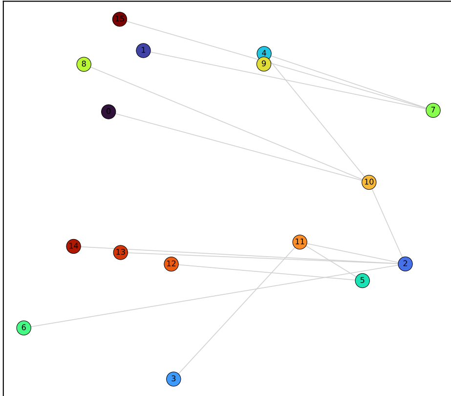
Llama layer 15/31 (PC var 17·13%)
