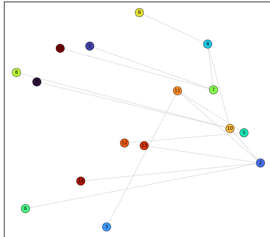
Qwen layer 20/35 (PC var 13·11%)
