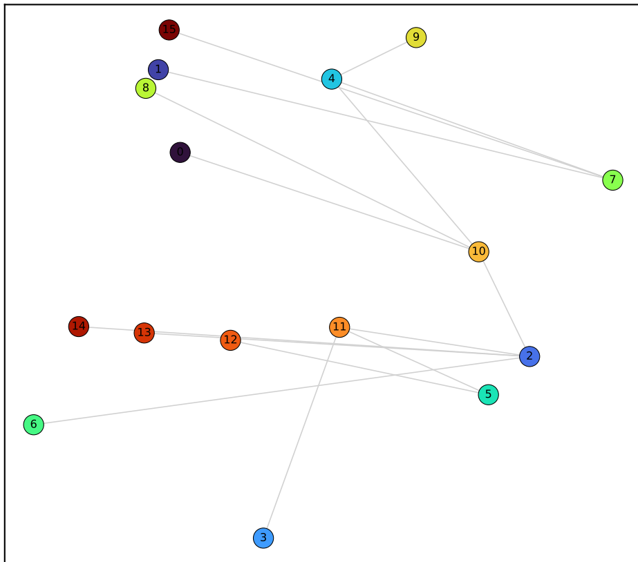
Llama layer 21/31 (PC var 16·13%)
