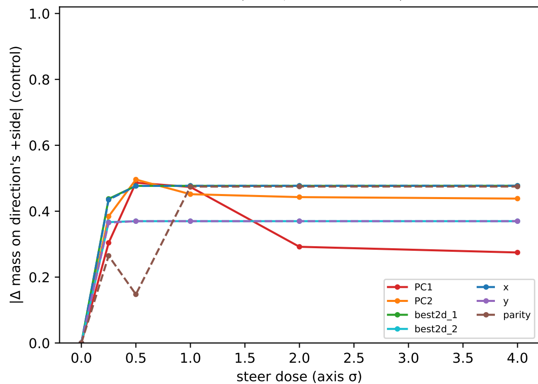
Llama ( L^*=30 , best2d-RSA=0.89)
