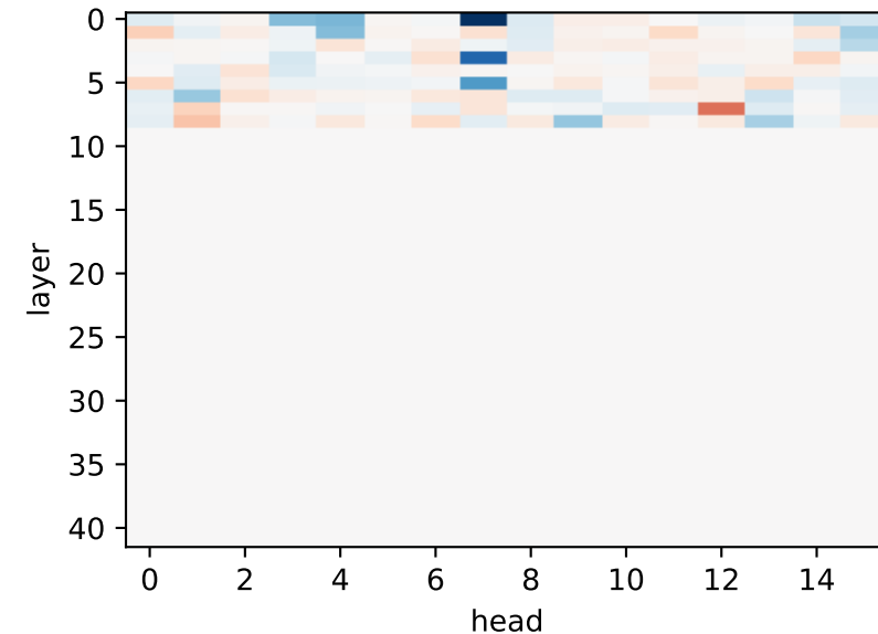
mode 7 ( \lambda 2.6 , pow 0.07)
