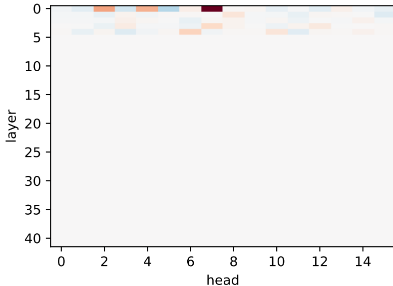
mode 6 ( \lambda 3.4 , pow 0.07)
