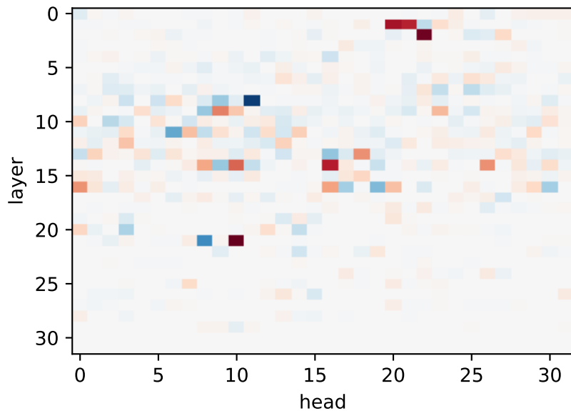
mode 4 ( \lambda 2.1 , pow 0.07)
