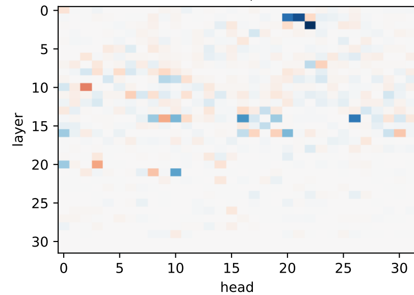
mode 7 ( \lambda 3.8 , pow 0.07)
