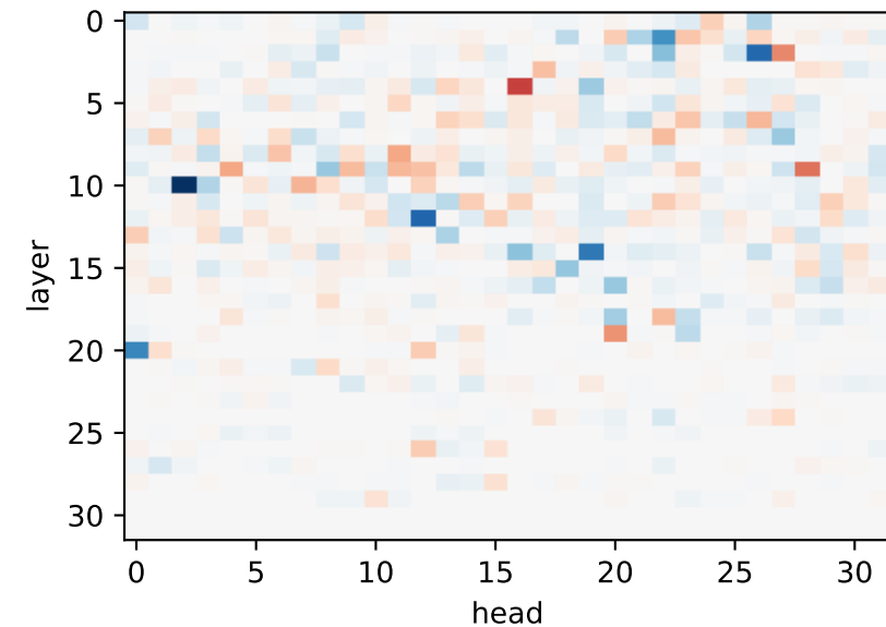
mode 7 ( \lambda 3.8 , pow 0.07)
