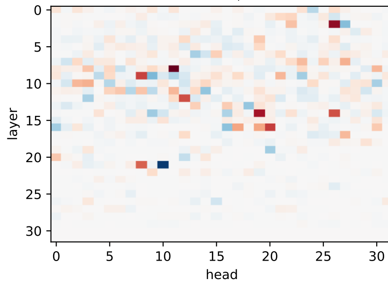
mode 12 ( \lambda 6.3 , pow 0.07)
