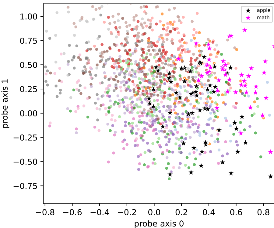
Llama L13 POST
